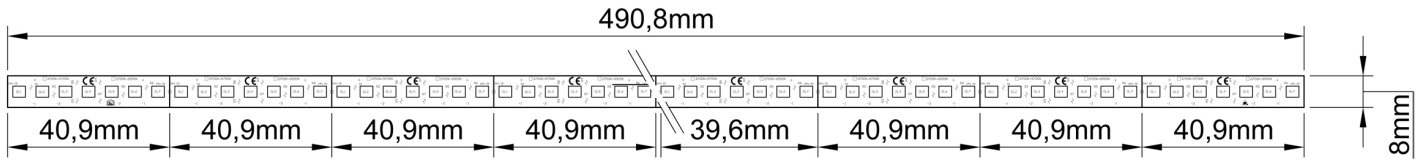
DISEGNO DIMENSIONALE ERI_115 DIMENSIONAL DRAWING ERI_115
