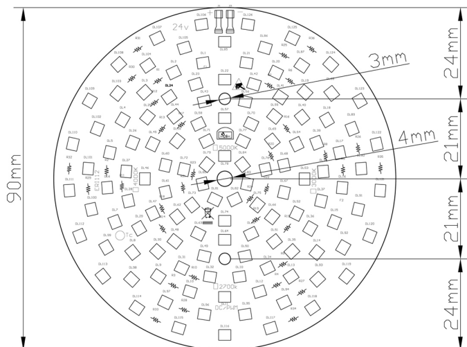
DISEGNO DIMENSIONALE DIMENSIONAL DRAWING
