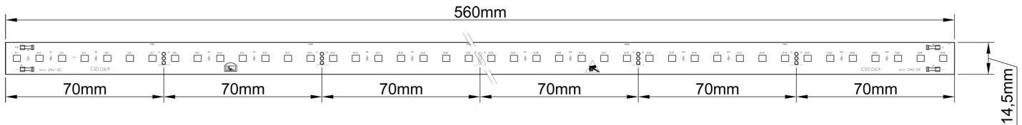
DISEGNO DIMENSIONALE ERI_064 DIMENSIONAL DRAWING ERI_064
