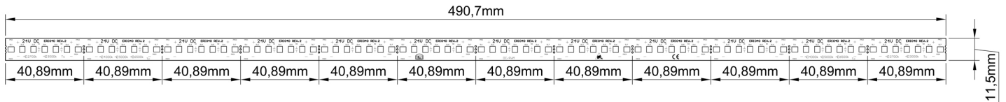
DISEGNO DIMENSIONALE ERI_040 DIMENSIONAL DRAWING ERI_040
